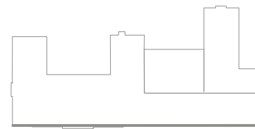
Фасад в осях 1-14
