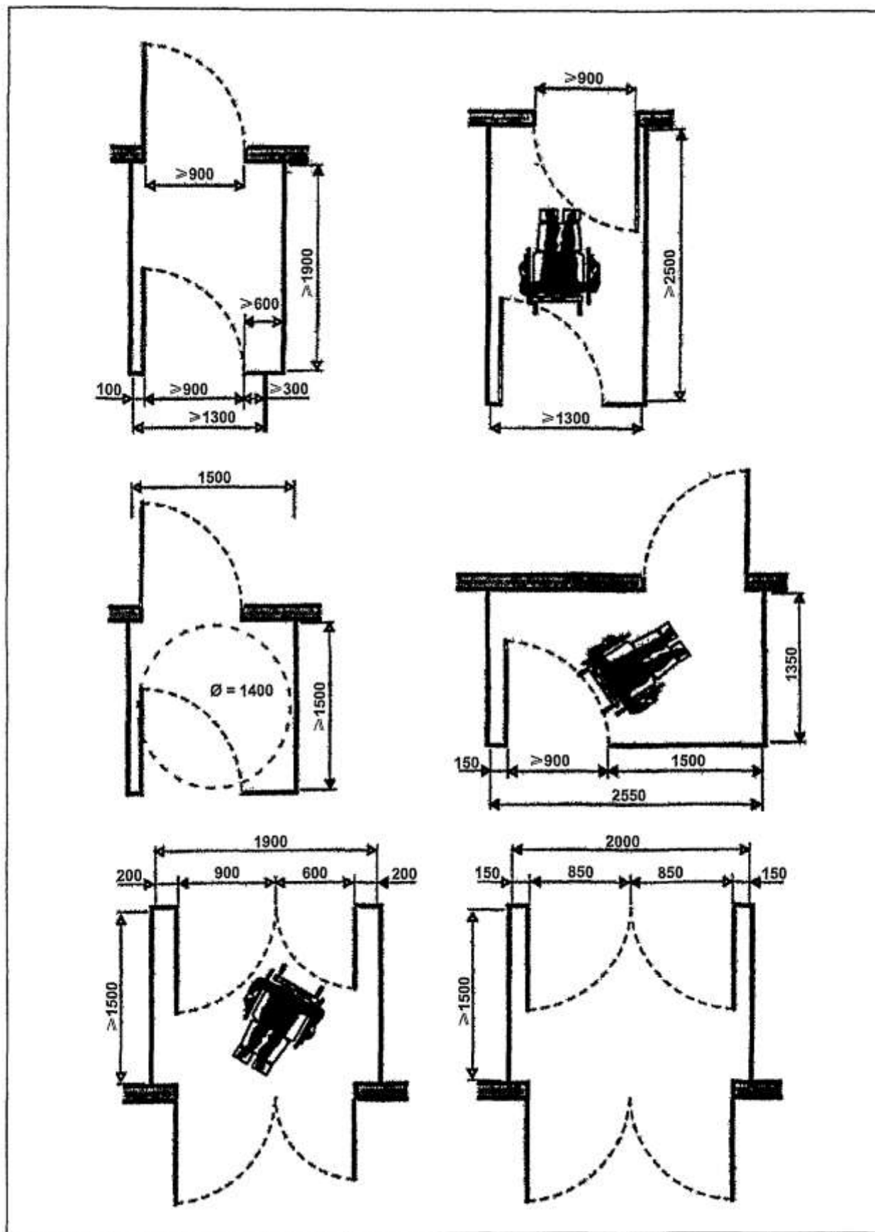
Рисунок Д.10 – Входные тамбуры
