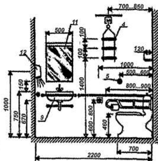
Разрез А-А
