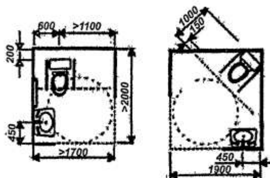
Примеры размещения санитарных приборов
